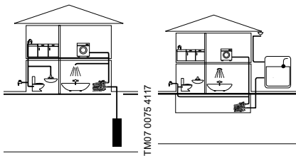
16-сүр. Скважинадан же резервуардан суу берүү
