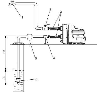
Նկար 9 Ջրիորից/հորատանցքից ջրի մատուցում
